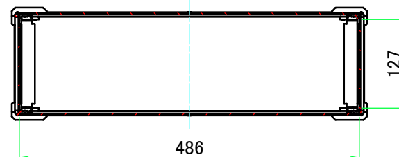
A-A ( 1 : 7.5 )
