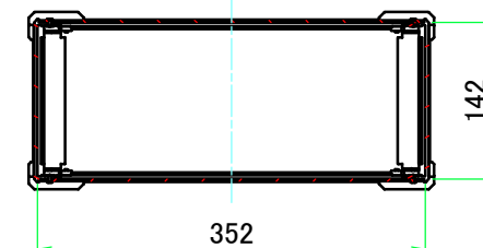
C-C ( 1 : 7.5 )
