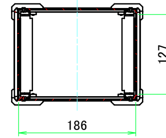
A-A (1:6)
