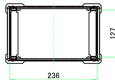
A-A (1:6)
