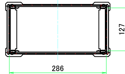
A-A ( 1 : 6.5 )
