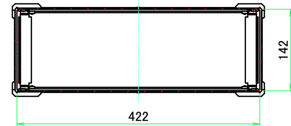
C-C ( 1 : 6.5 )
