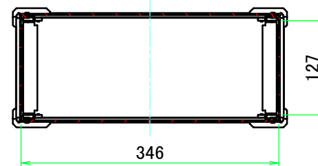
A-A (1:7)
