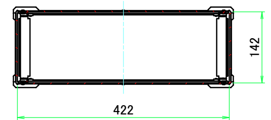
C-C ( 1 : 7.5 )
