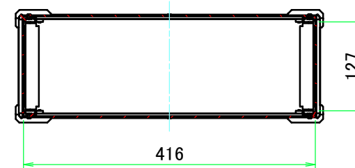
A-A ( 1 : 7.5 )
