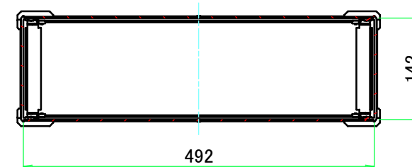
C-C ( 1 : 7.5 )
