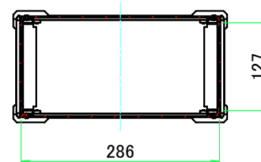
A-A ( 1 : 7.5 )
