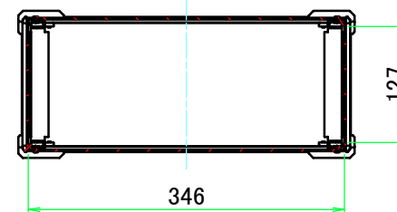
A-A ( 1 : 7.5 )
