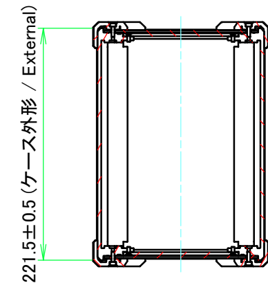
D-D (1:5)
