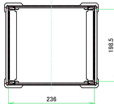
A-A (1:5)
