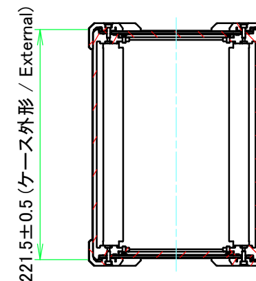
D-D (1:5)
