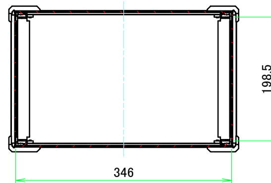
A-A (1:6)
