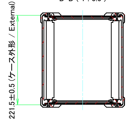
D-D ( 1 : 5.5 )
