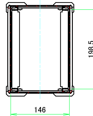
A-A ( 1 : 5.5 )
