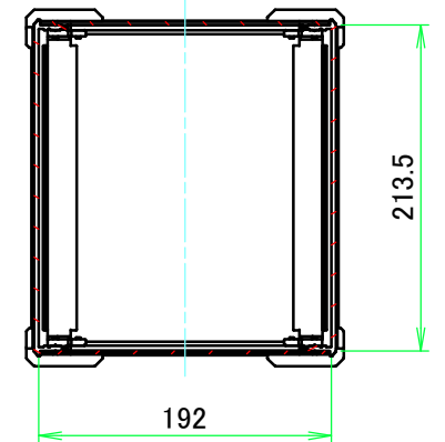
C-C ( 1 : 5.5 )
