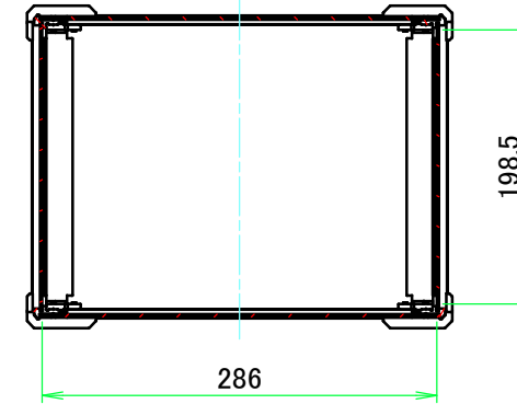
A-A (1:6)
