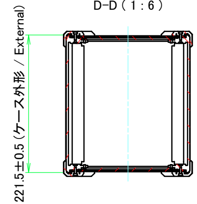
D-D (1:6)
