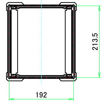
C-C ( 1 : 6.5 )
