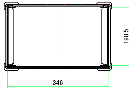
A-A ( 1 : 6.5 )
