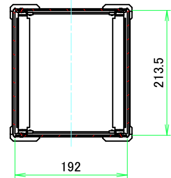
C-C ( 1 : 6.5 )
