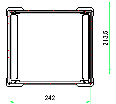
C-C ( 1 : 5.5 )
