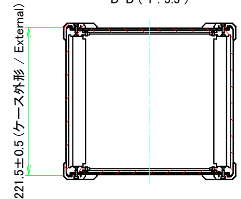
D-D ( 1 : 5.5 )
