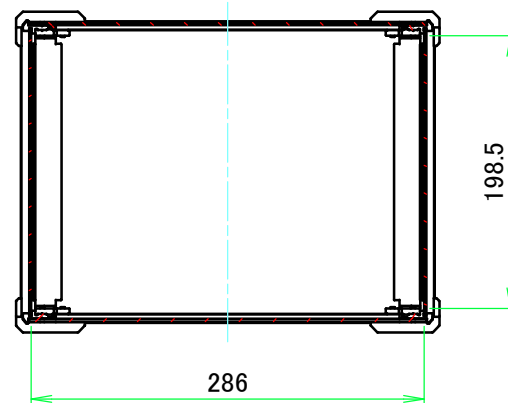
A-A ( 1 : 5.5 )
