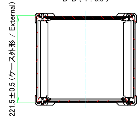
D-D ( 1 : 5.5 )
