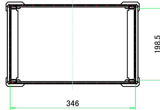
A-A ( 1 : 6.5 )
