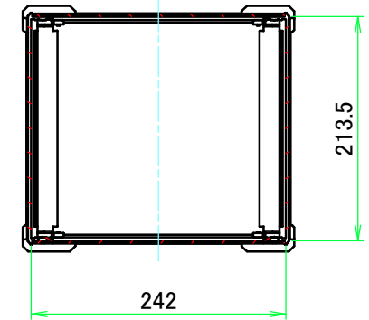
C-C ( 1 : 6.5 )
