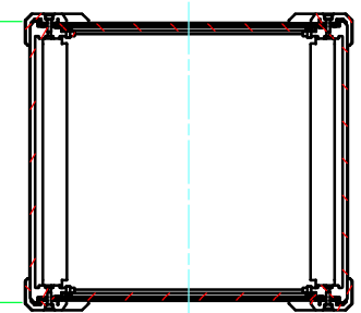
D-D (1:6.5)
