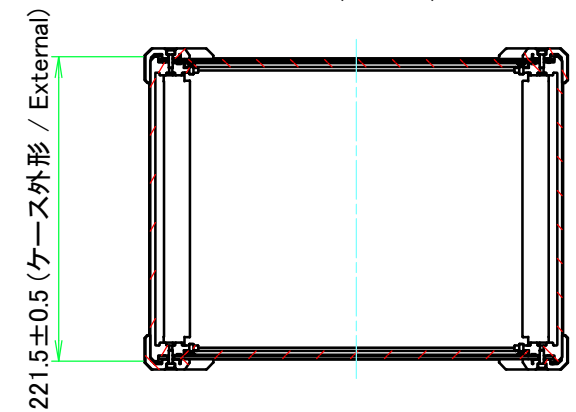
D-D ( 1 : 5.5 )
