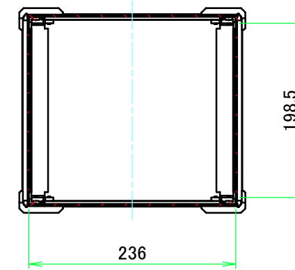
A-A (1:6)
