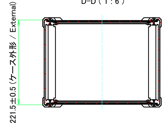
D-D (1:6)
