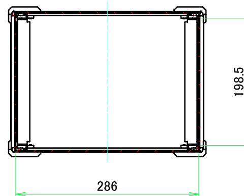
A-A (1:6)
