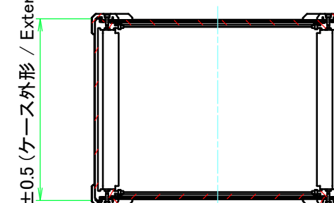
D-D (1:6.5)
