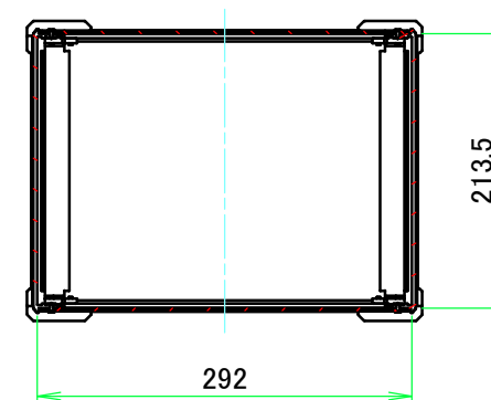
C-C ( 1 : 6.5 )
