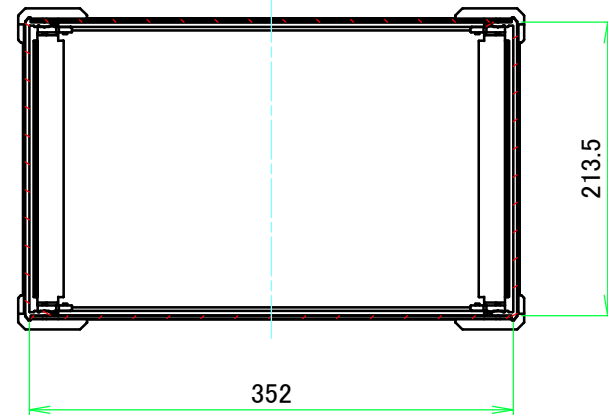
C-C ( 1 : 5.5 )
