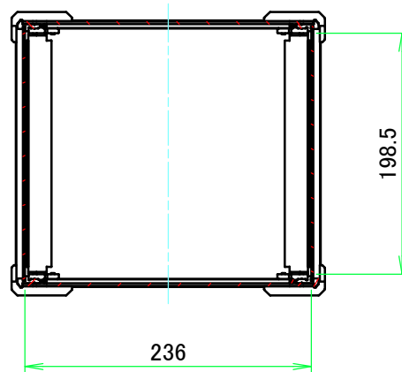
A-A ( 1 : 5.5 )
