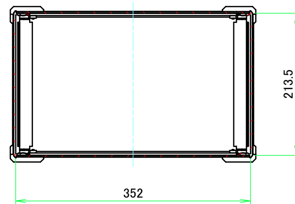
C-C ( 1 : 5.5 )
