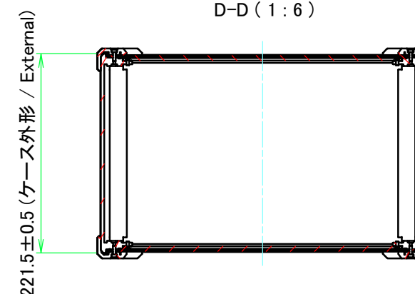
D-D (1:6)
