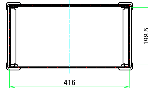
A-A (1:7.5)
