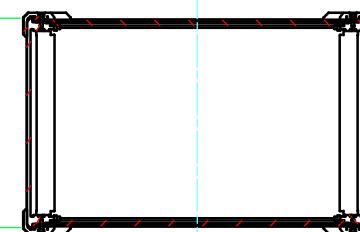
D-D (1:8)
