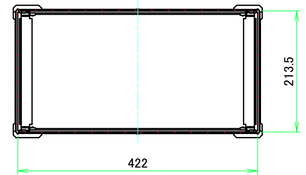
C-C ( 1 : 6.5 )
