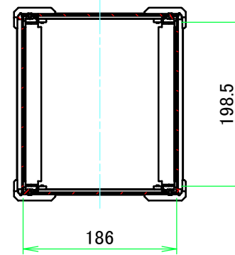
A-A ( 1 : 6.5 )
