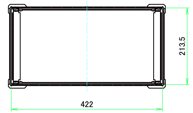
C-C ( 1 : 6.5 )
