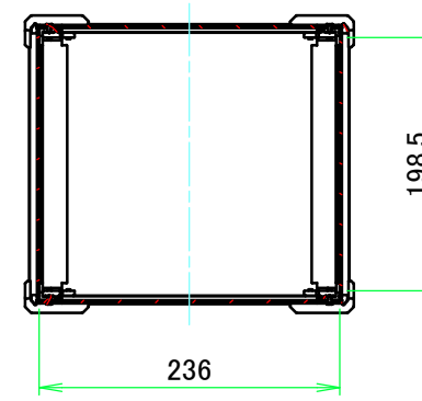
A-A ( 1 : 6.5 )
