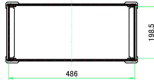
A-A ( 1 : 8.5 )
