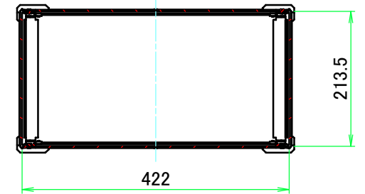
C-C ( 1 : 8.5 )
