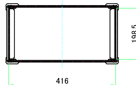
A-A (1:9)
