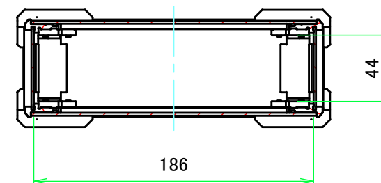
A-A ( 1:3.5 )
