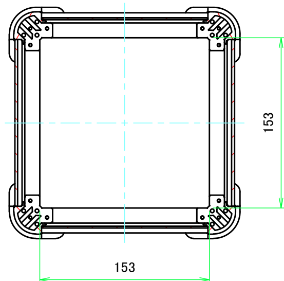
B-B ( 1:3.5 )
