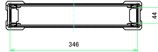
A-A ( 1:5 )
