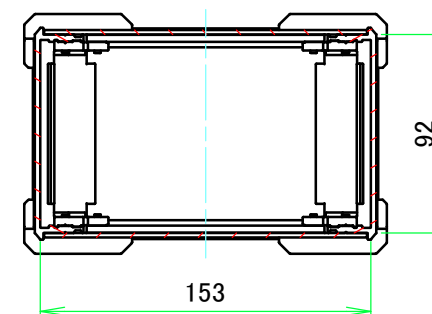
C-C ( 1 : 3.5 )
