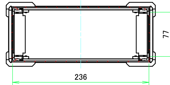
A-A (1:4)
