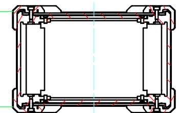
D-D (1:4)
