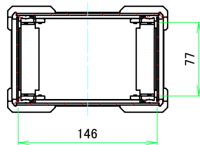
A-A (1:4)
