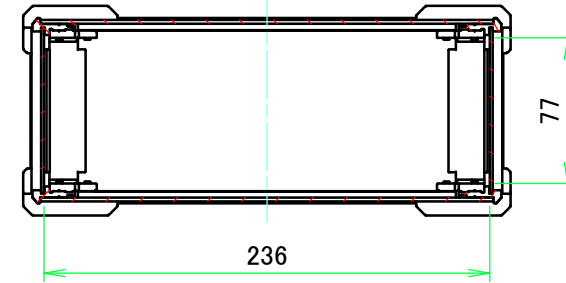
A-A (1:4)
