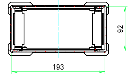
C-C ( 1 : 4.5 )
