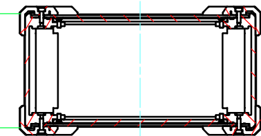
D-D ( 1 : 4.5 )
