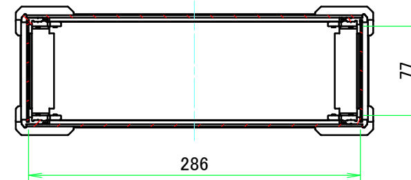
A-A (1:4.5)
