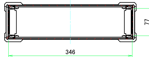
A-A (1:5)
