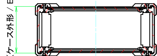
D-D (1:5)
