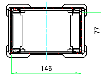
A-A ( 1 : 4.5 )
