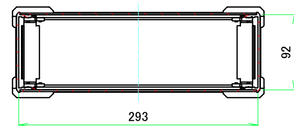
C-C ( 1 : 4.5 )
