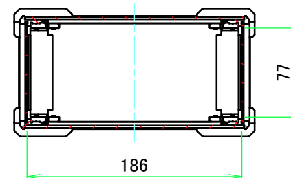
A-A (1:4.5)
