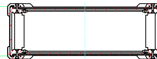
D-D ( 1 : 4.5 )
