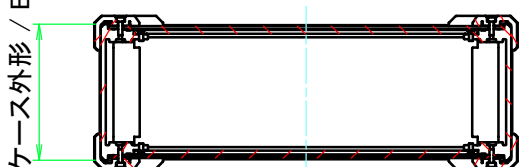
D-D ( 1 : 5.5 )
