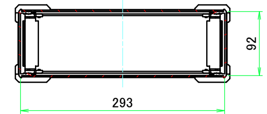
C-C ( 1 : 5.5 )
