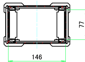
A-A (1:5)
