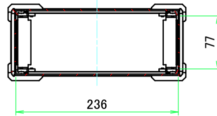
A-A ( 1 : 5.5 )
