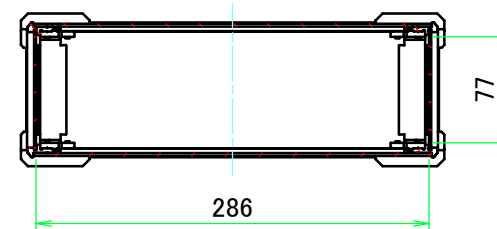
A-A ( 1 : 5.5 )
