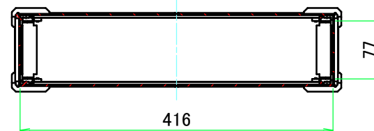
A-A (1:7)
